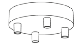
KRM574FVBTERP 4 hole ø 120mm H 25mm
